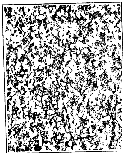
F. Coarse silt (1/32-1/16mm.), x 18
