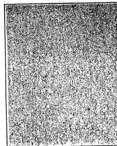
H. Fine silt (1/256-1/64 mm.), x 6.3
