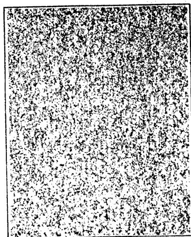
F. Coarse silt (1/32-1/16 mm.), x 6.3
