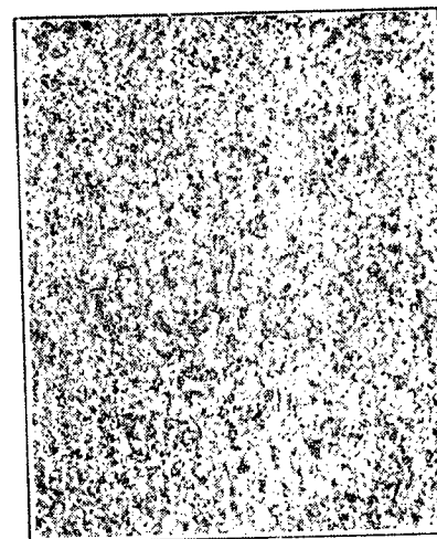
H. Fine silt (1/256-1/64 mm.), x 18
