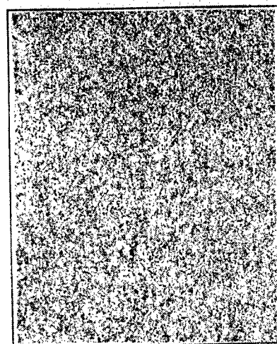
G. Medium silt (1/64-1/32 mm.), x 6.3
