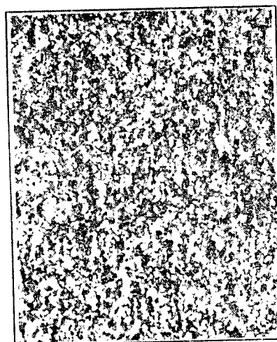
G. Medium silt (1/64-1/32 mm.), x 18
